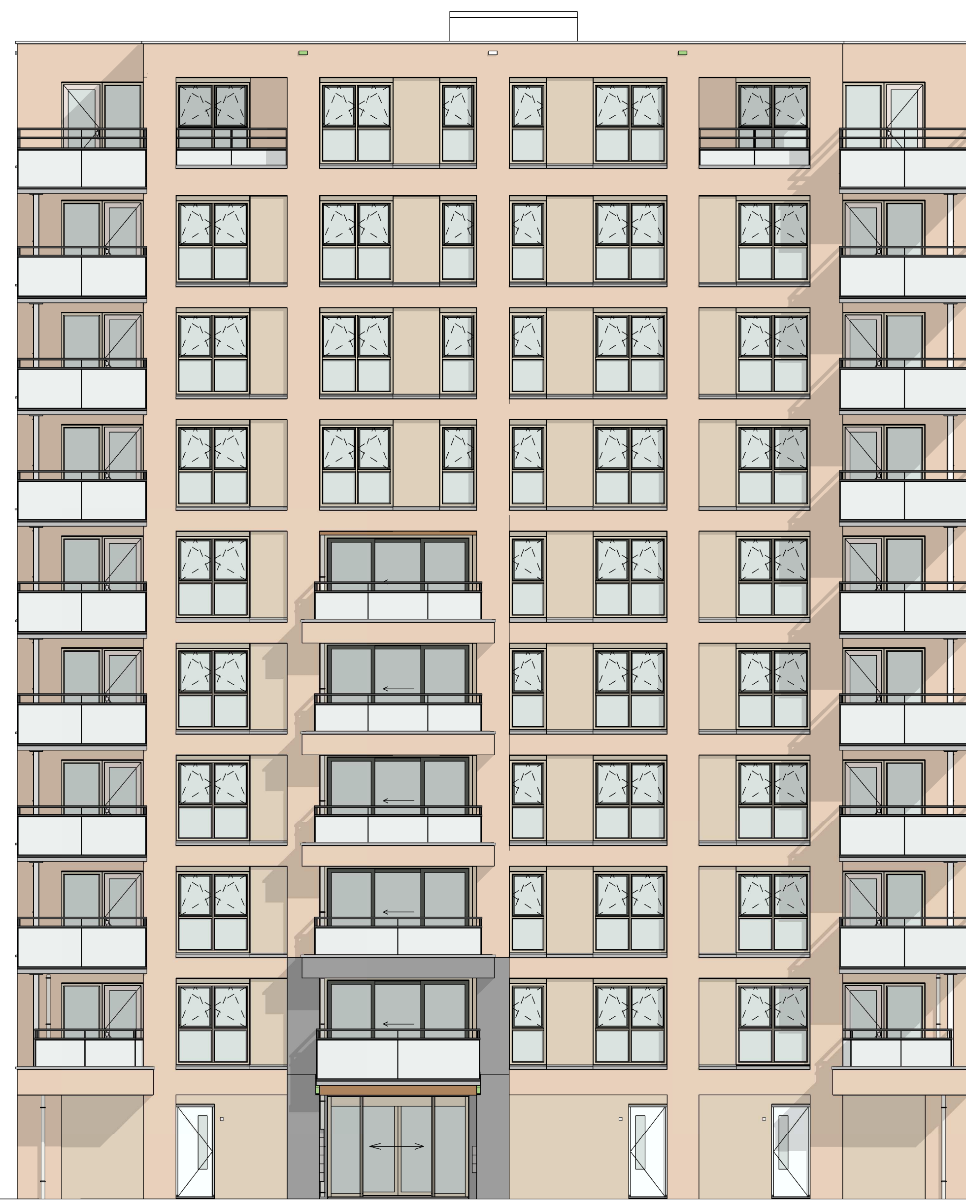
voorgevel
