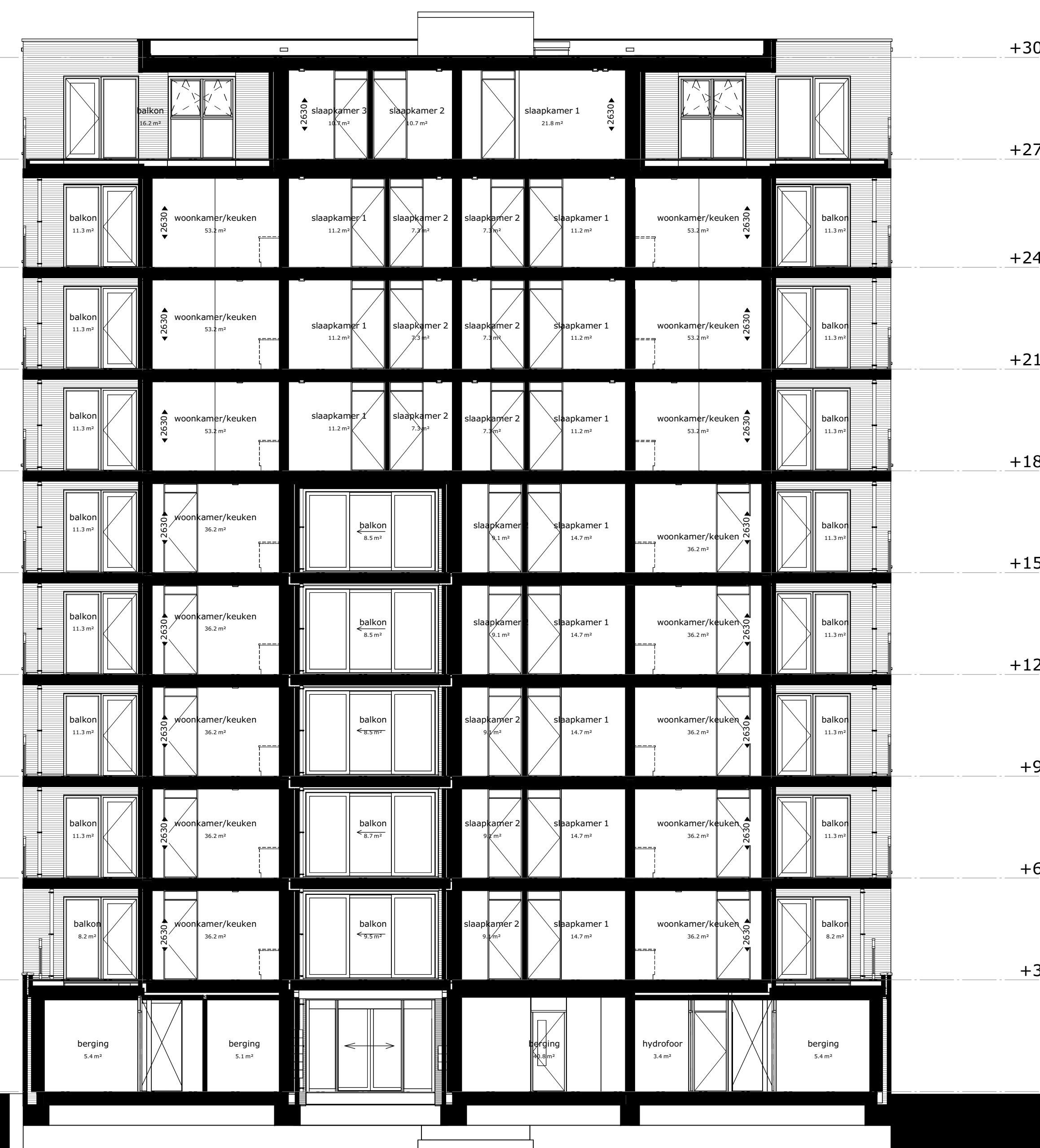
doorsnede B
