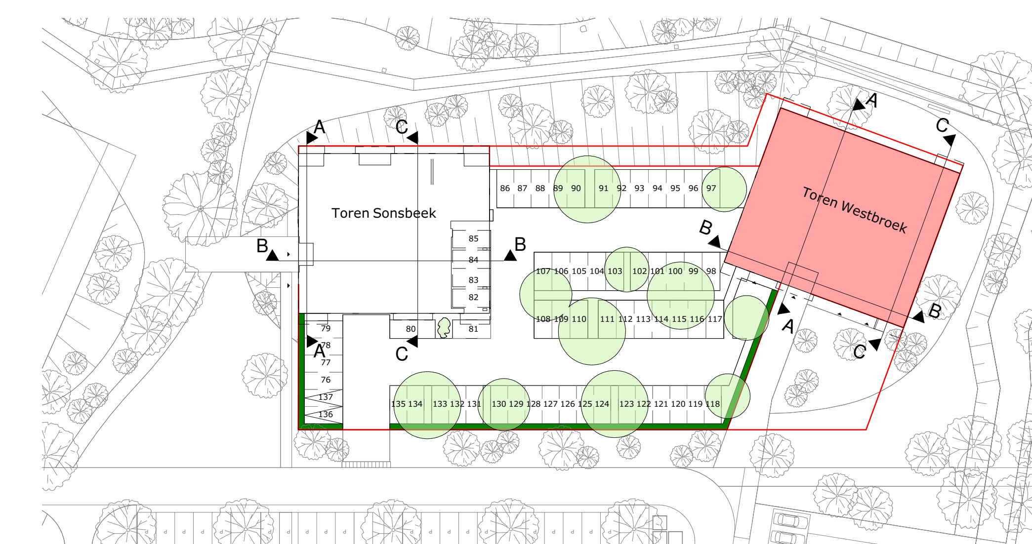
situatie
