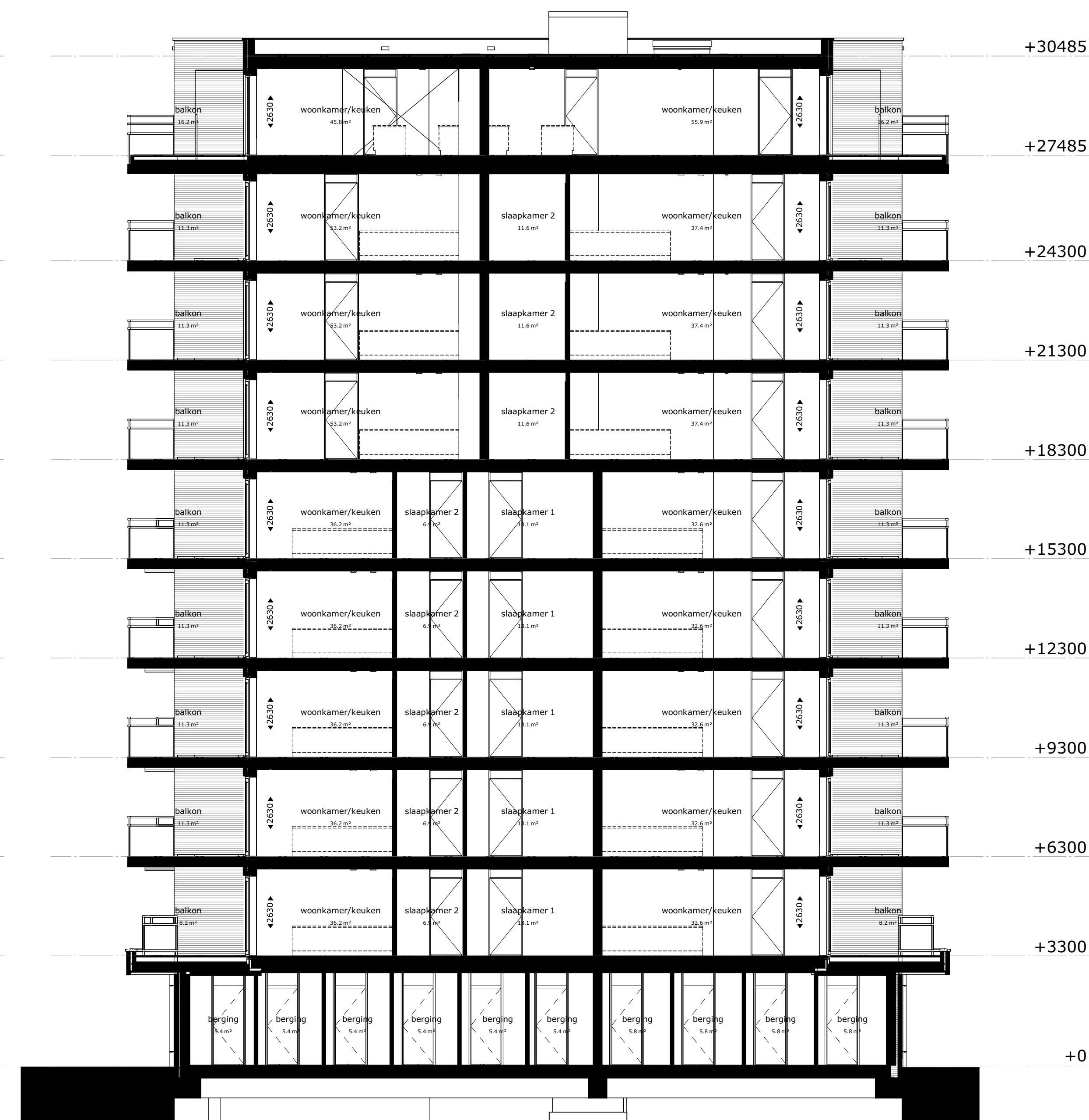
doorsnede C
