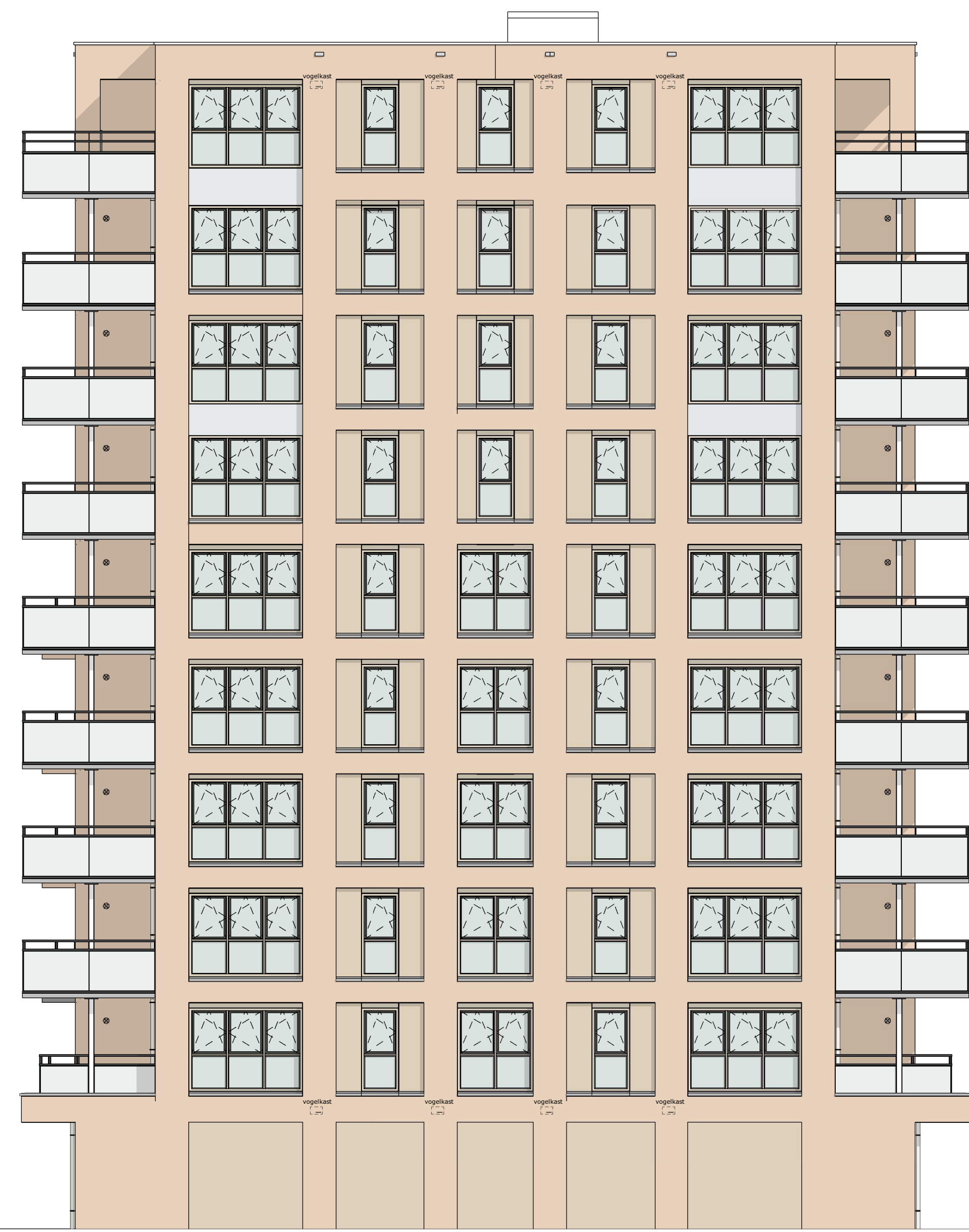
rechter zijgevel
