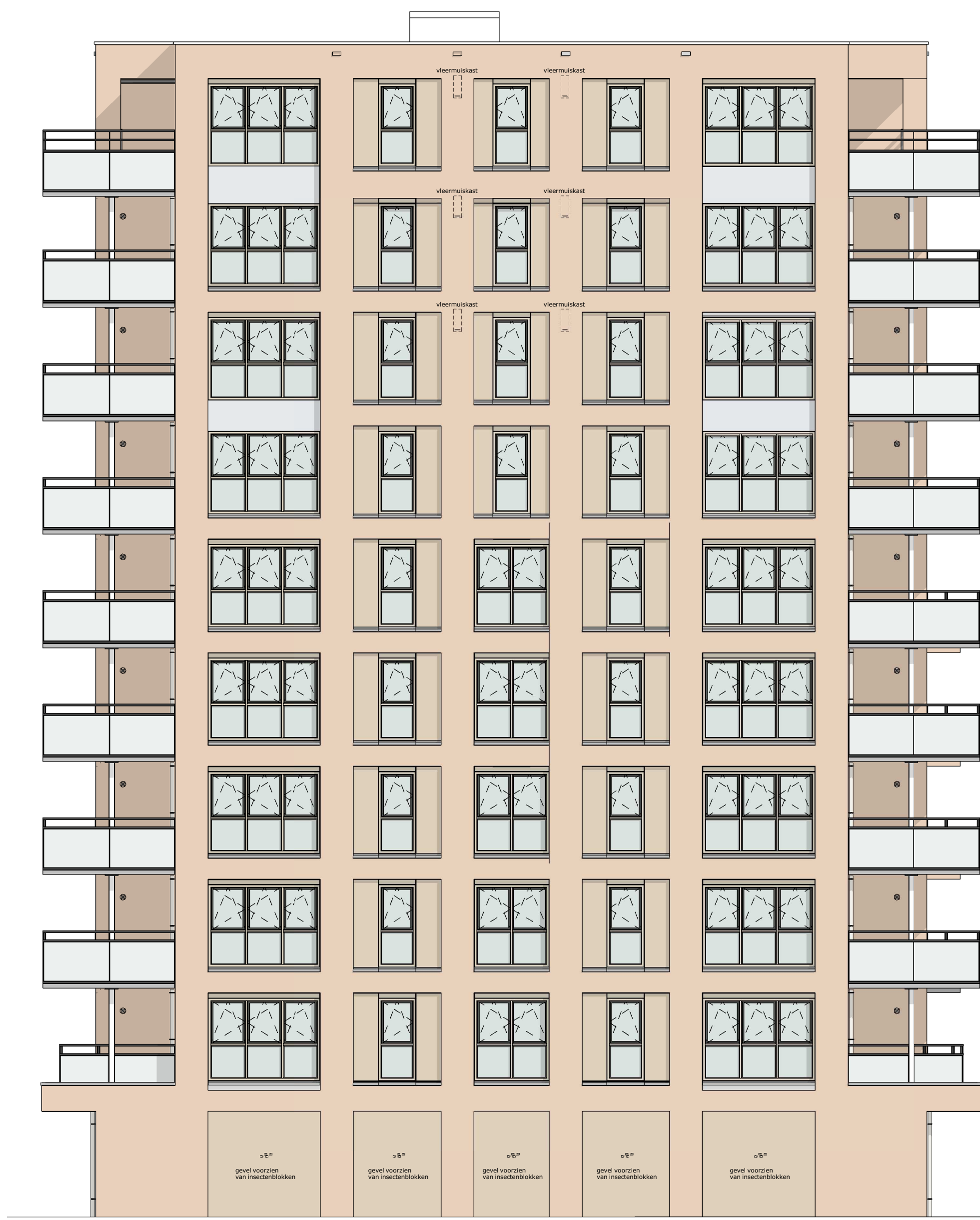
linker zijgevel
