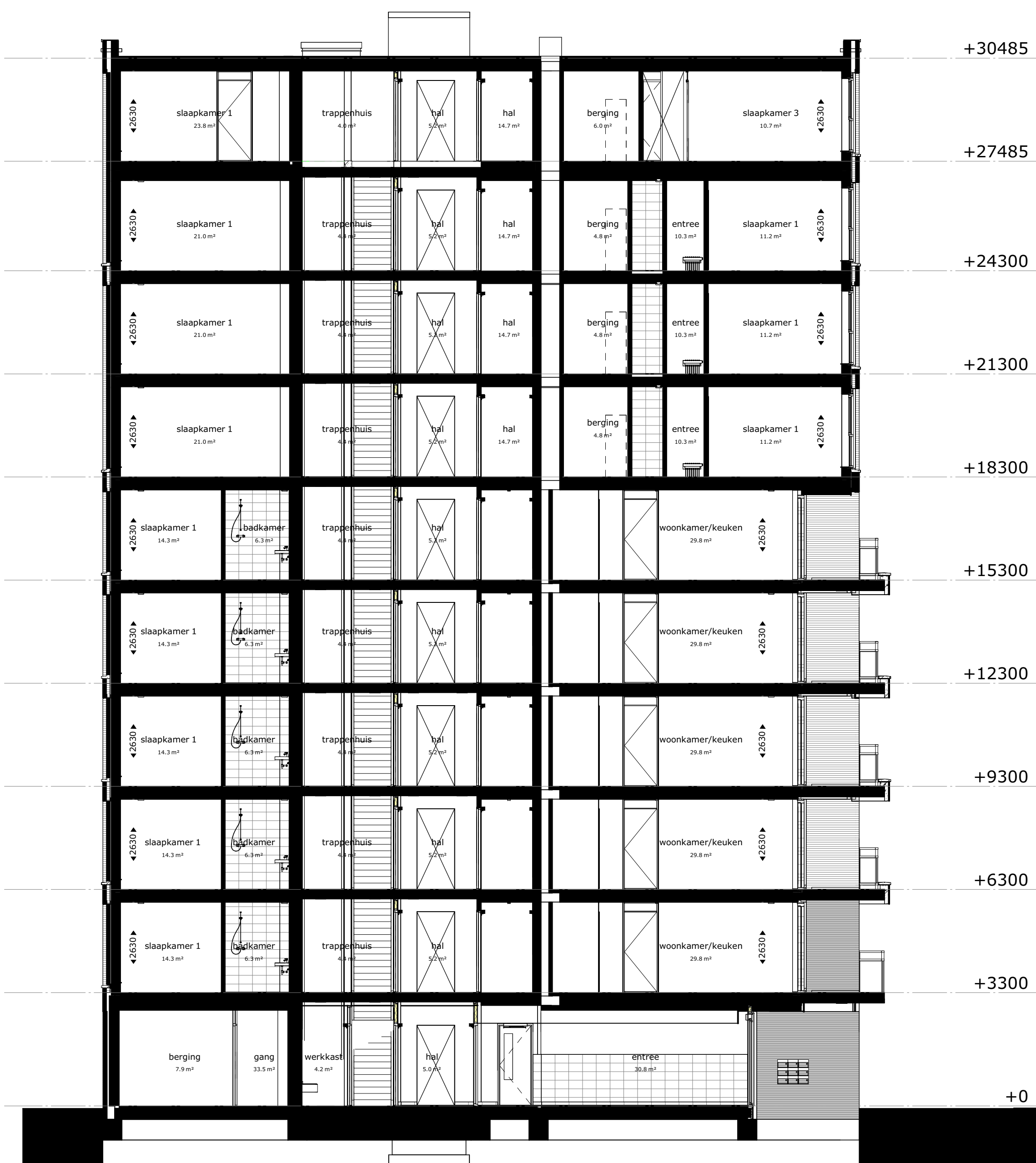
doorsnede A
